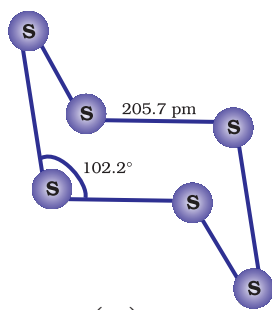
चित्र 7.5 (ख) साइक्लो S_6 रूप संरचनाएँ
