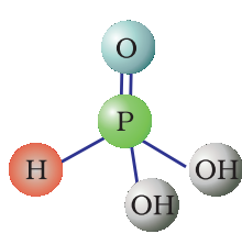
H_3PO_3 आर्थोफॉस्फोरस अम्ल
