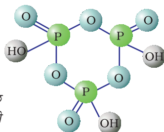
(HPO_3)_3 साइक्लोट्राइमेटाफॉस्फोरिक अम्ल
